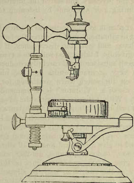
Fig. 32A. Vibrator.
